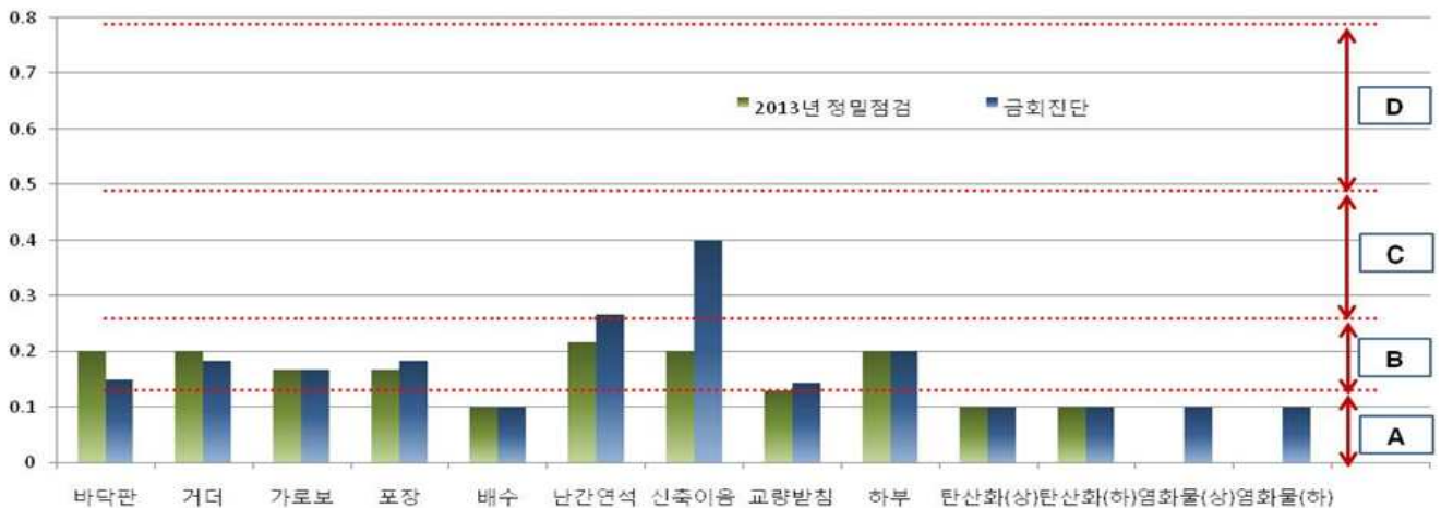
【그림 4.3.1】 기 점검 결과와의 부재별 상태평가 결과 비교(대구)
